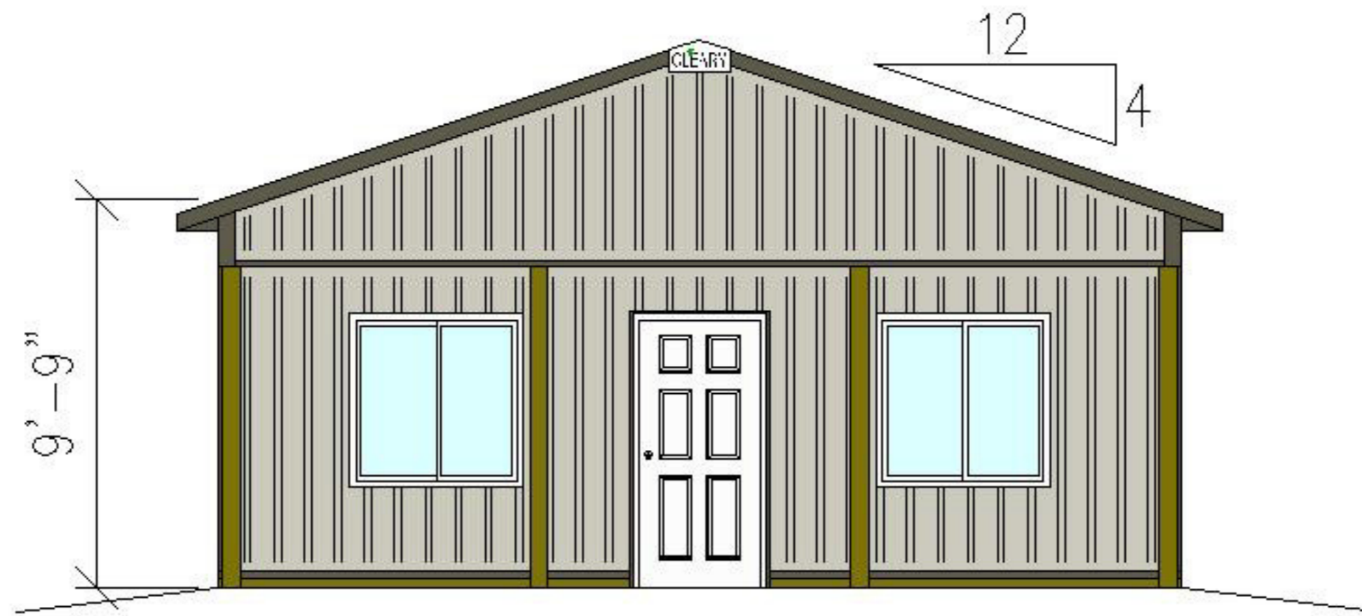
END ELEVATION
