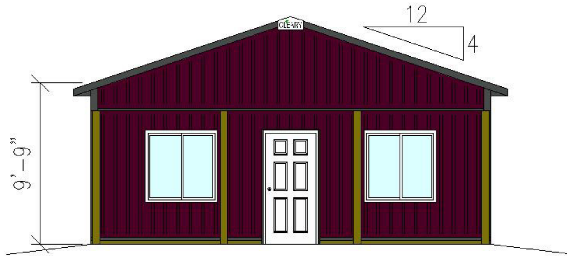
END ELEVATION
