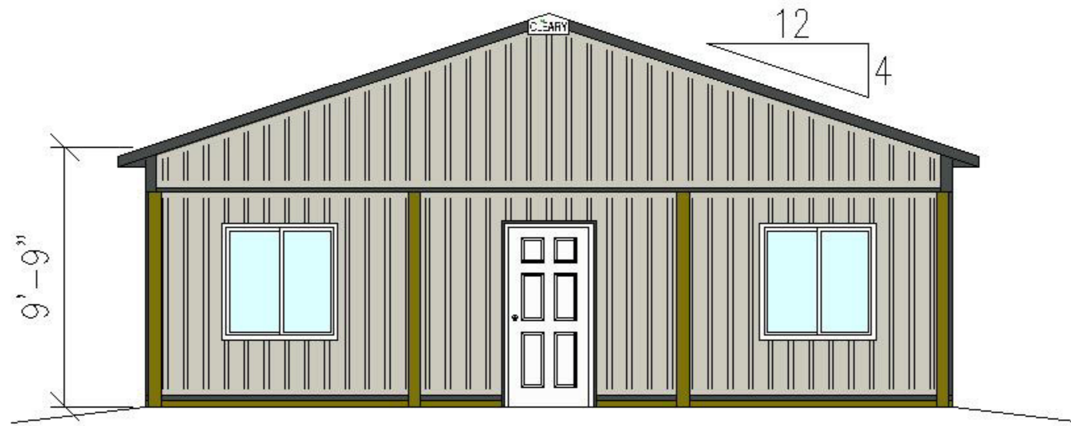
END ELEVATION
