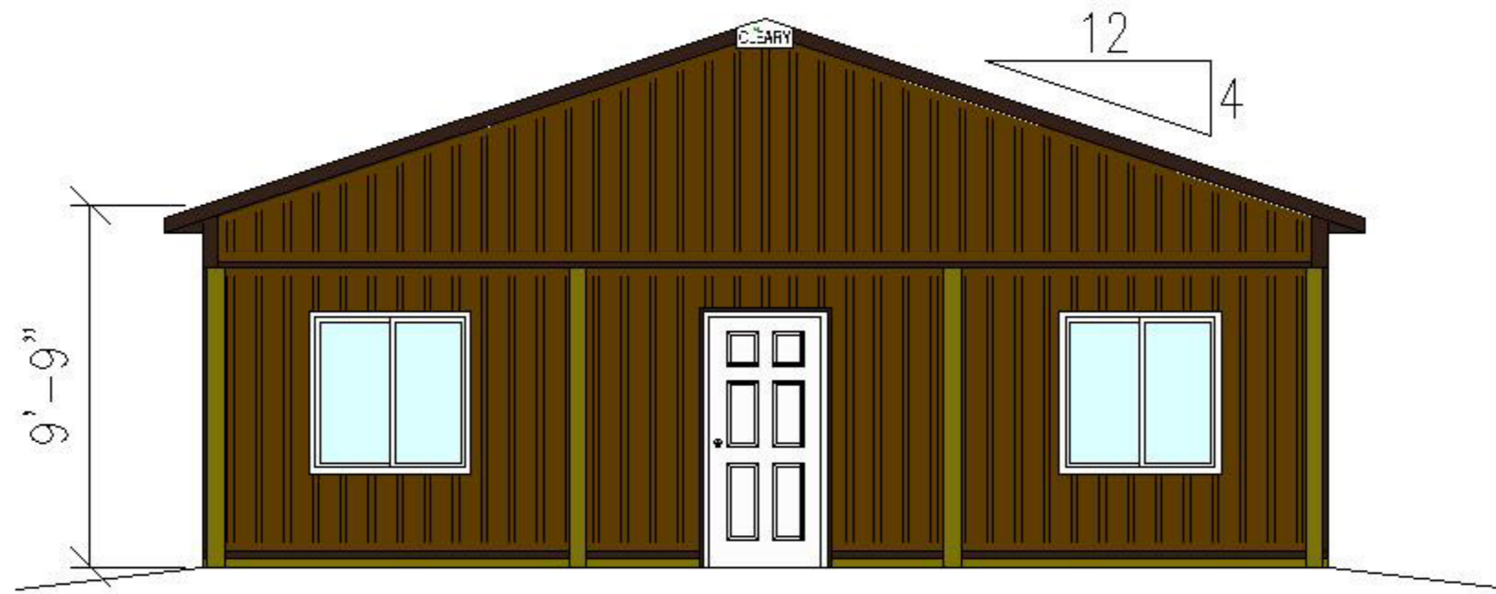
END ELEVATION
